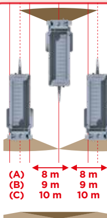
Largeurs de croisement (variables selon la matière épandue) : (A) 8 m (standard) (B) 9 m avec couteaux cuillères (C) 10 m avec plateaux d'épandage
